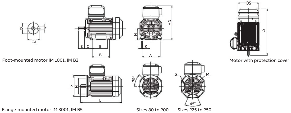
Flange-mounted motor IM 3001, IM B5
